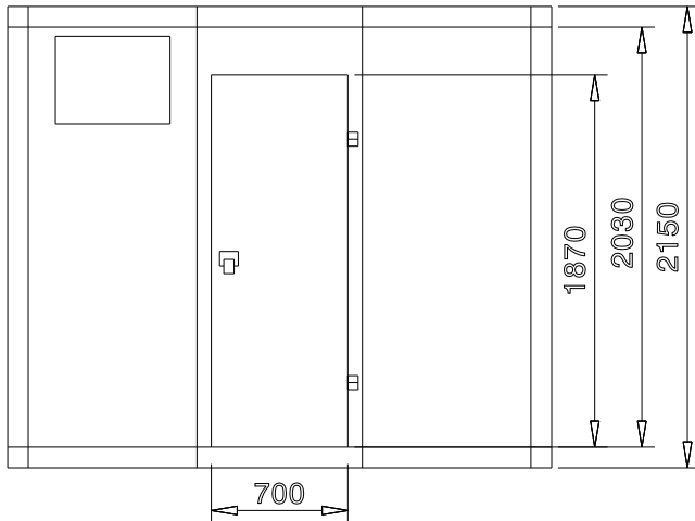
Zij aanzicht
