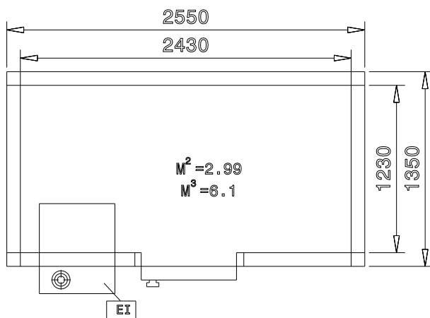
Zij aanzicht
